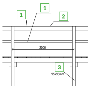
ALÇADO LONGITUDINAL ÉLEVATION LONGITUDINALE LONGITUDINAL ELEVATION
