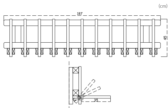
CUBA DE LAVAGEM REF. 2357 | BAC DE LAVAGE | WASH TUB
